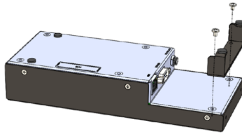
[Fig. 3] Removing bracket
